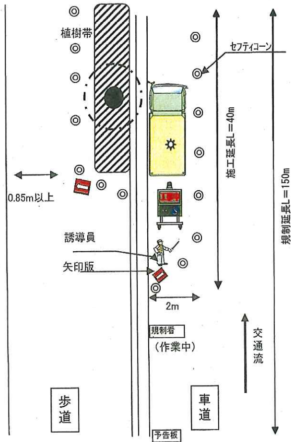
標準図
